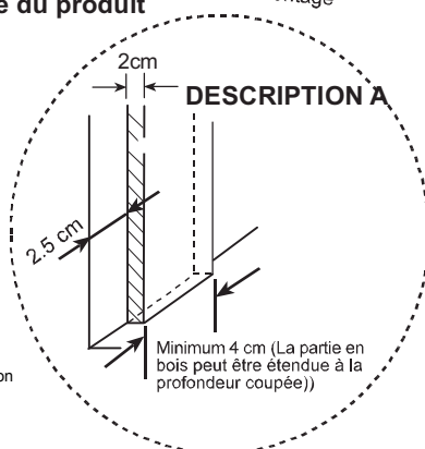
Vis de montage
